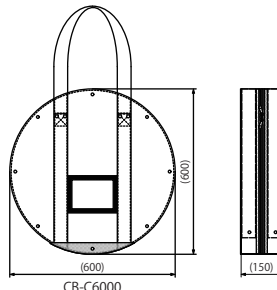
【外形寸法図】
